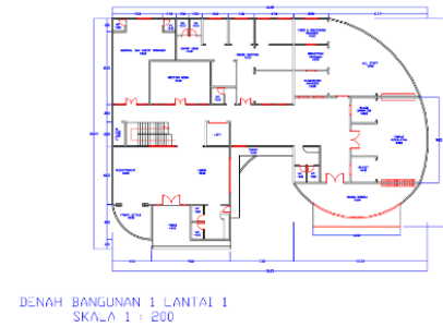
Gambar 14 Denah bangunan 2
